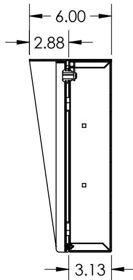
SECTION A-A
